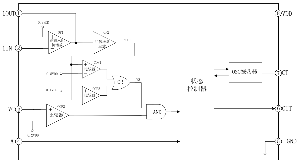
图 5-1. EG4003 结构框图
